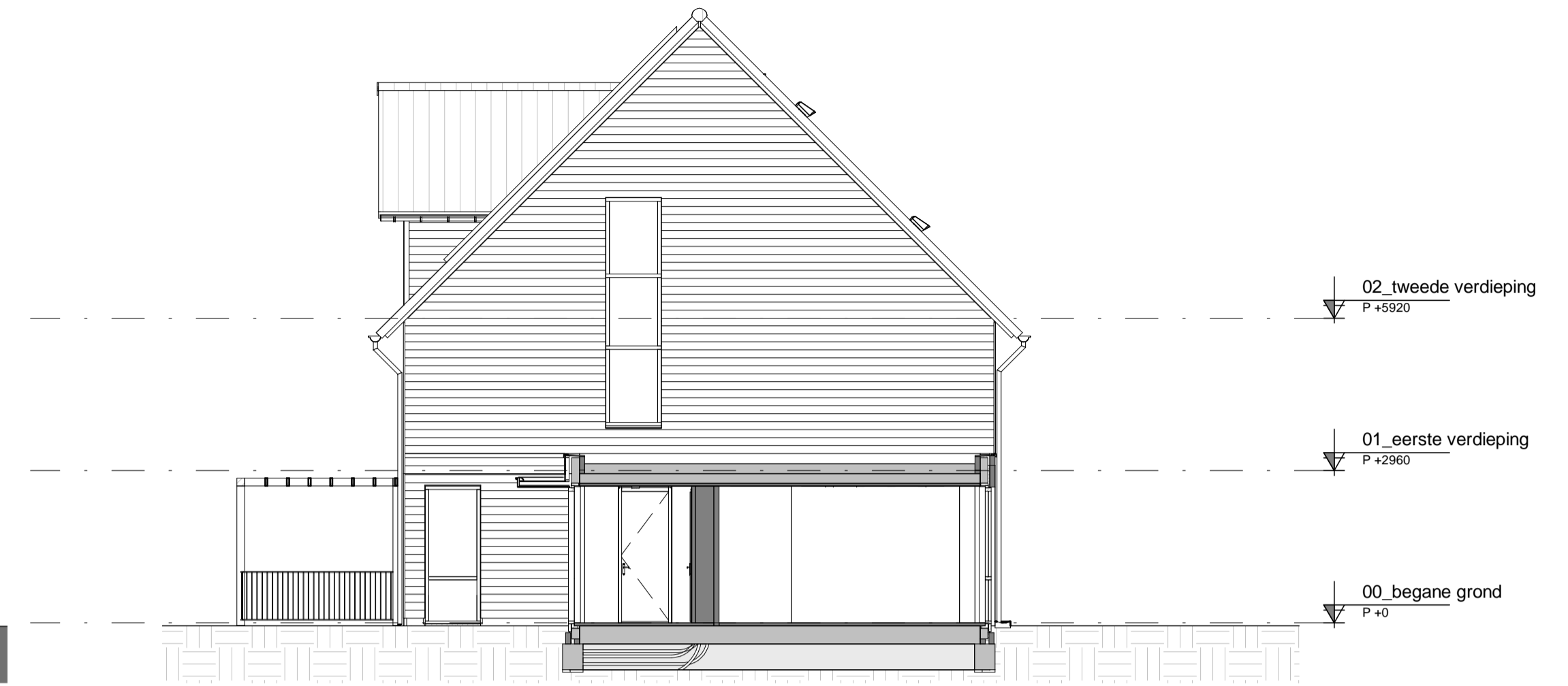
Doorsnede B.A
